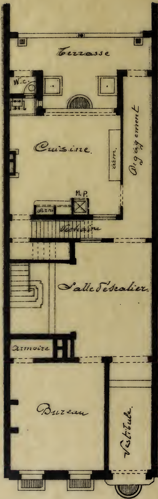
Plan du rez-de-chaussée.
